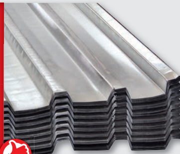
IBR 0.4 FH/0.686m 3.6m SKU: 612 324.95 4.8m SKU: 616 432.95 6m SKU: 620 467.95
